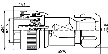
NRW-24※-PM□
