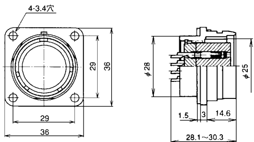
NRW-28※-RF
