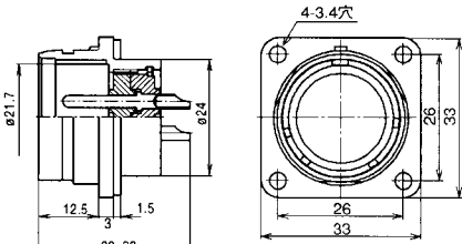
NRW-24※-RM
