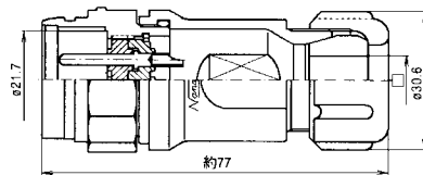
NRW-24※-AdM□
