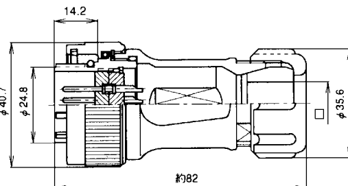
NRW-28※-PM
