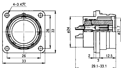
NRW-24※-RF
