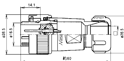
NRW-20※-PM□
