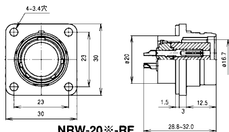
NRW-20※-RF
