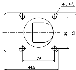
NJW-24用Lザ(座)
