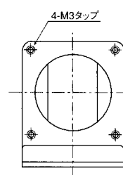
NJW-20用Lザ(座) ※使用方法は7ページ参照
