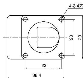
NJW-20用Lザ(座) ※使用方法は7ページ参照
