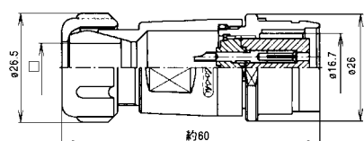
NRW-20※-AdF□
